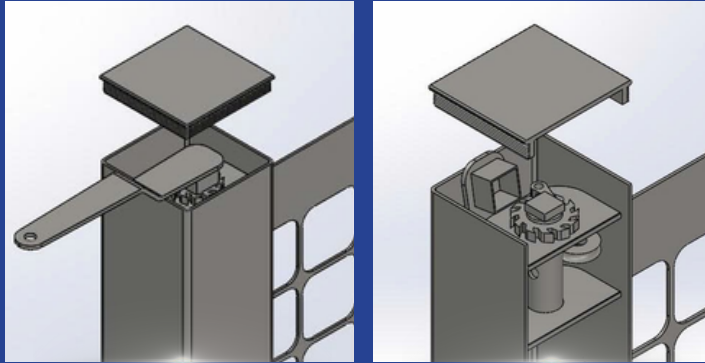
Khi gắn tay quay căng lưới
